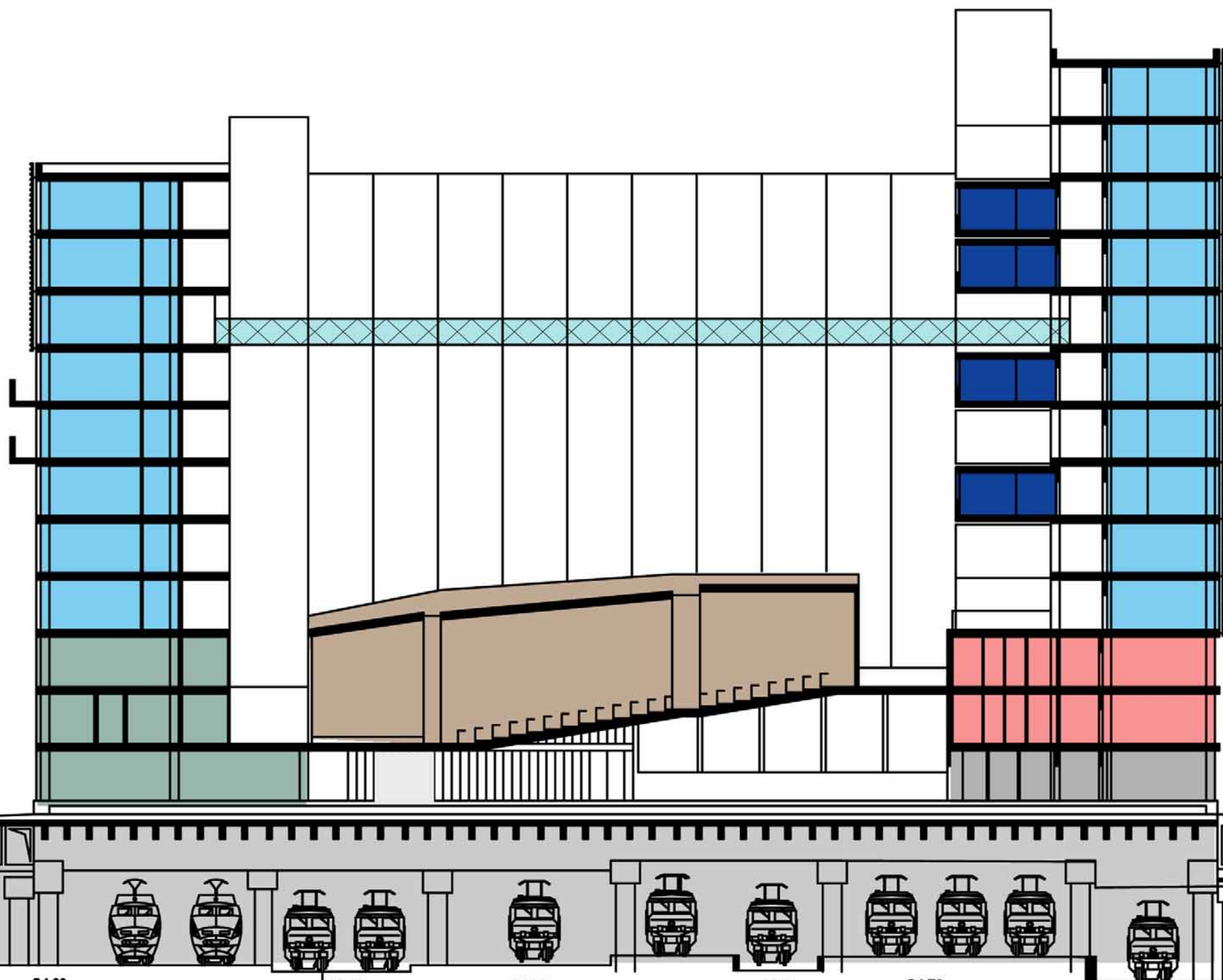
coupe transversale 1/200
