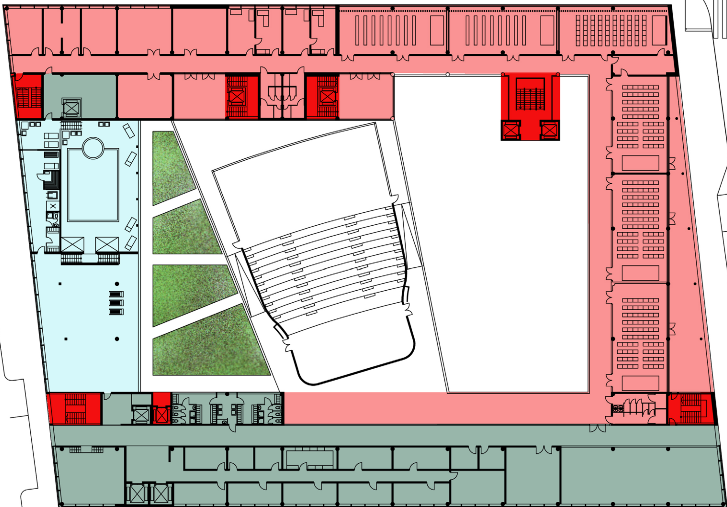
plan de 1er étage 1/250
